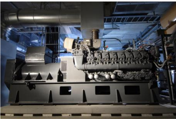
Die Notstromdiesel-Anlage
